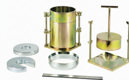
Ensemble de Moules CBR
