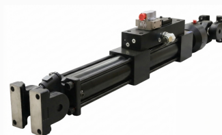
Système d'actionneurs servo hydrauliques. 500kN
