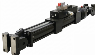
Système d'actionneurs servo hydrauliques. 500kN
