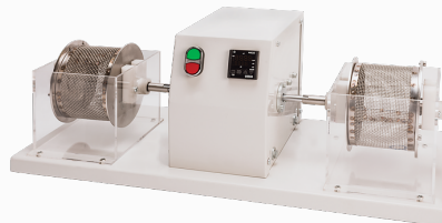
Appareil de durabilité de clatement
