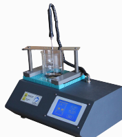
Appareil automatique de point de ramollissement (Anneau et
