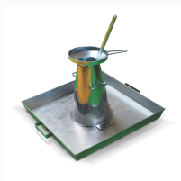
Cône d'Abrams complet
