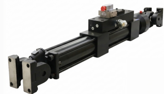
Servo Hidrolik Quasi Static Aktüatör Sistemi. 500kN
