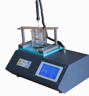
Otomatik Yumuşama Noktası Denev Cihazı
